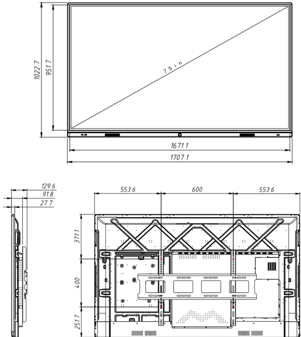
外观尺寸图
