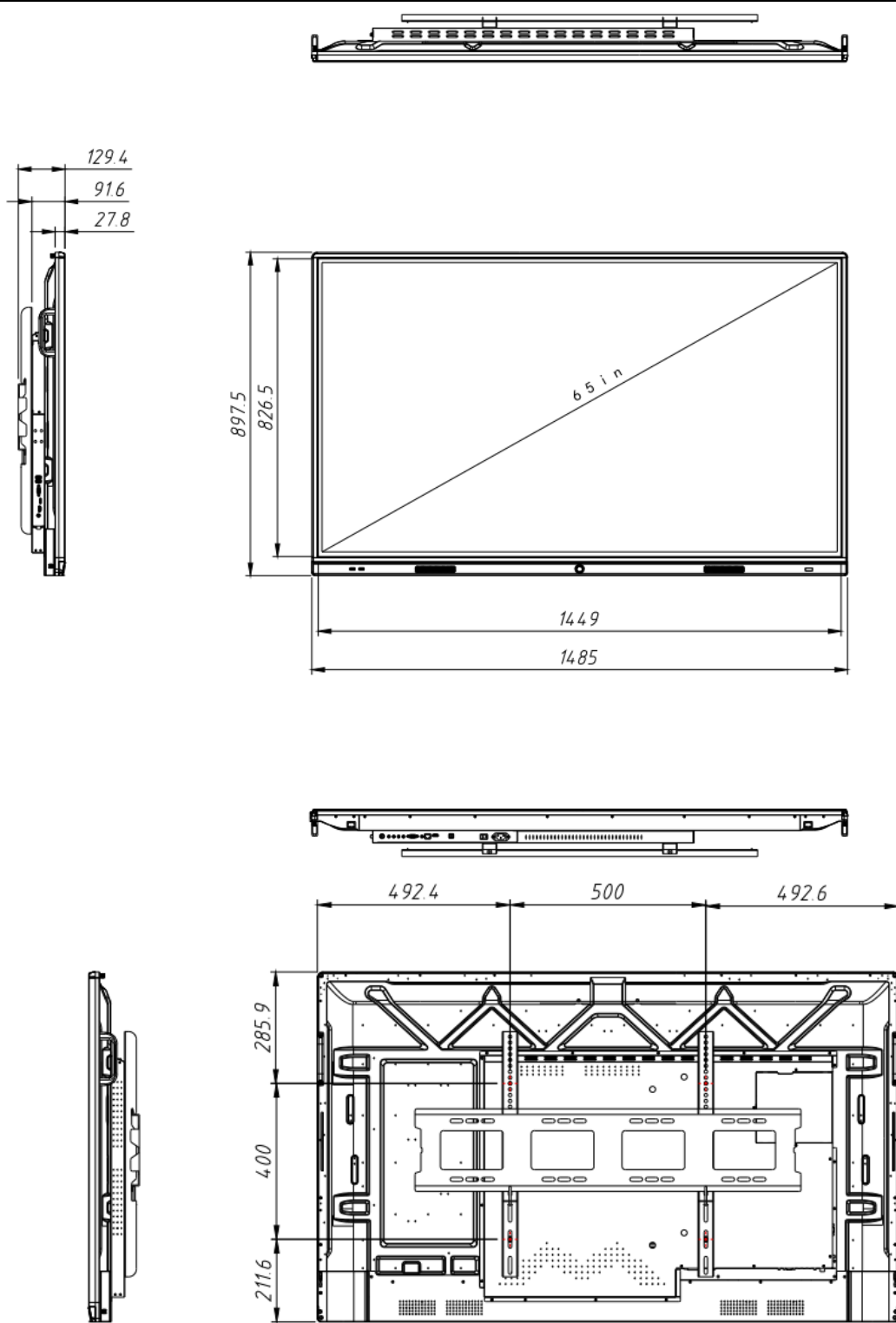
外观尺寸图
