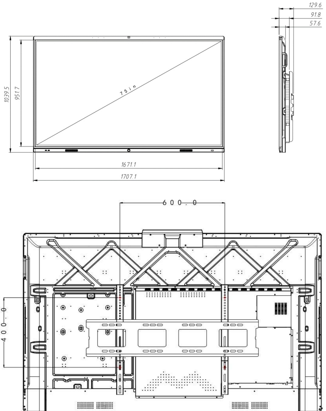
外观尺寸图
