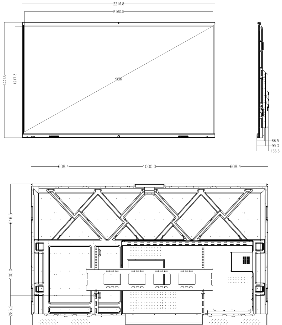
外观尺寸图
